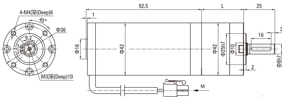
M向视图 (View M)
